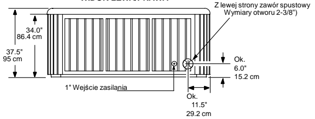
WIDOK LEWA/PRAWA
