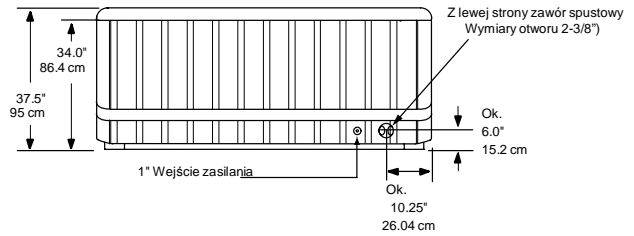
WIDOK LEWA/PRAWA
